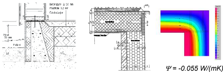
Figure 6 linear thermal conductivity \Psi \leq 0,01 \text{ W/(mK)} , sources: SINTEF Byggforsk, PHI, ProKlima
